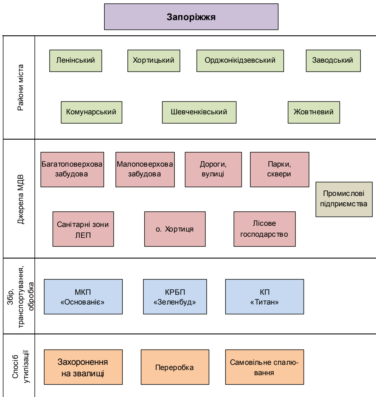
Рисунок 1.1. Умовна схема структури обігу деревинних відходів у місті
