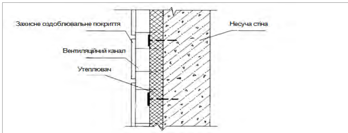
Рисунок 7.1.4. Утеплення стін за методом «керамічний вентиляований фасад»
