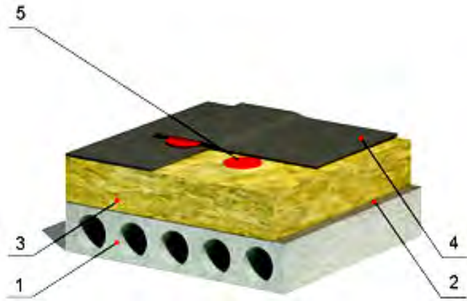
Рисунок 7.1.5. Структура утеплення дахового перекриття
