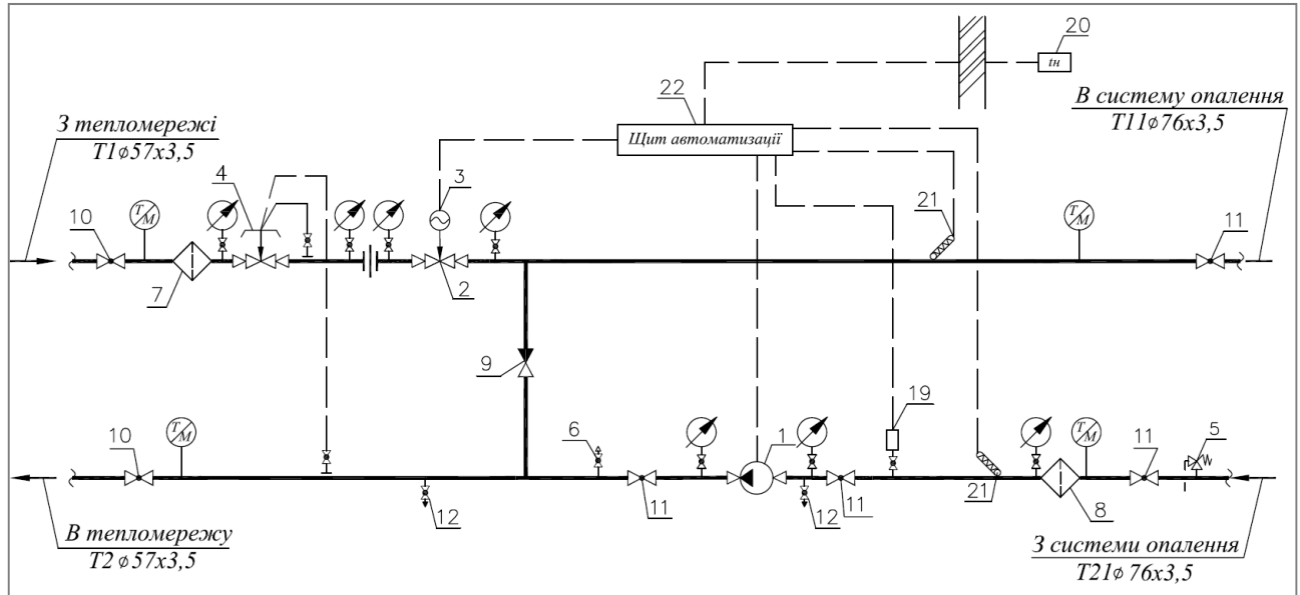
Рисунок С.1. Типова схема теплового пункту із залежним підключенням абонента
