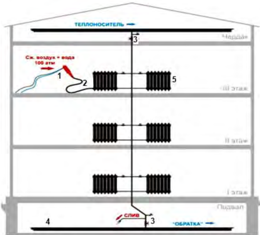
Рисунок 7.1.3. Схема очищення на прикладі 3-х поверхової будівлі.
