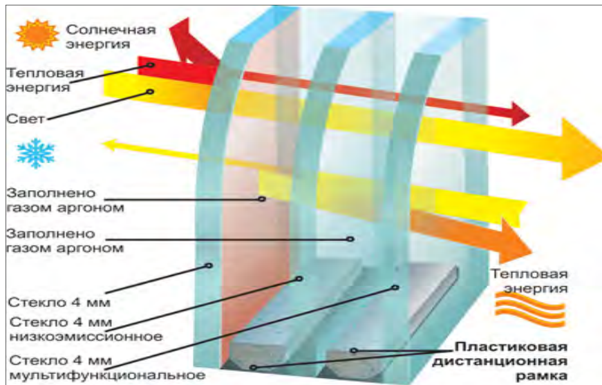
Рисунок 7.1.8. Енергозберігаючий склопакет
