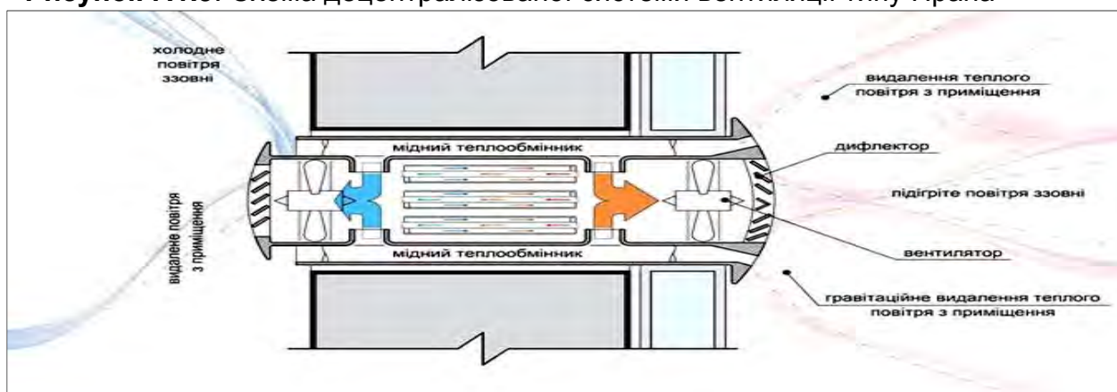
Рисунок 7.1.9. Схема децентралізованої системи вентиляції типу Прана
