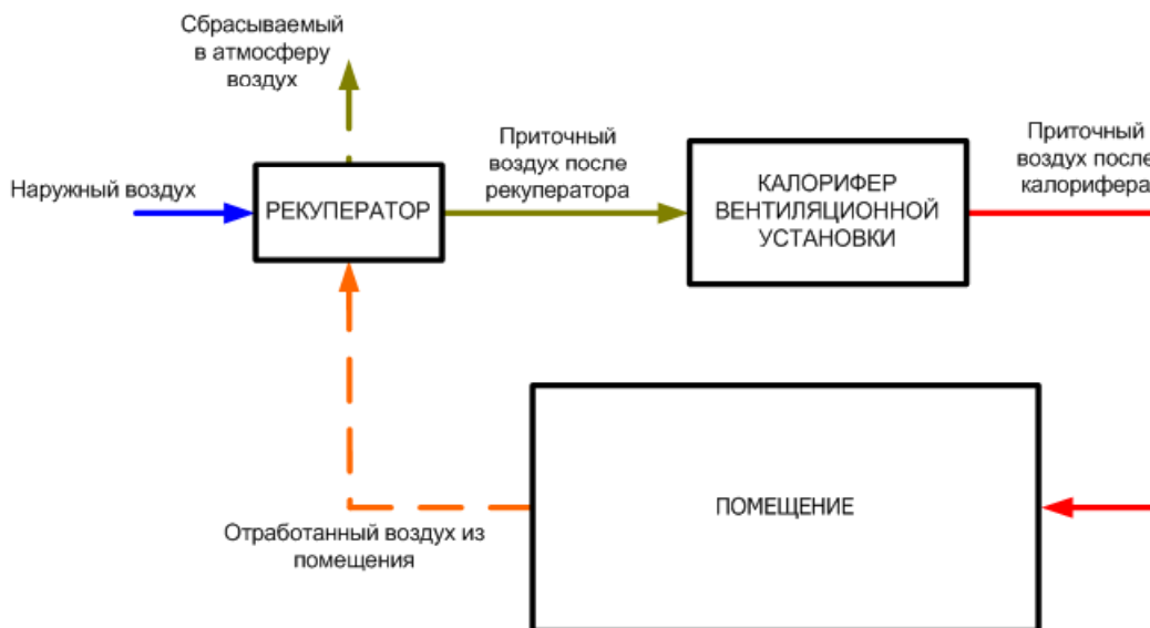
Рисунок D.1. Типова схема роботи системи рекуперації теплової енергії
