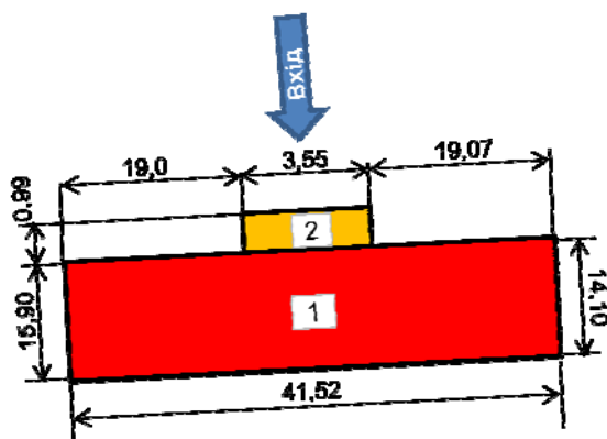
Рисунок 3.1. План забудови адміністративної будівлі
