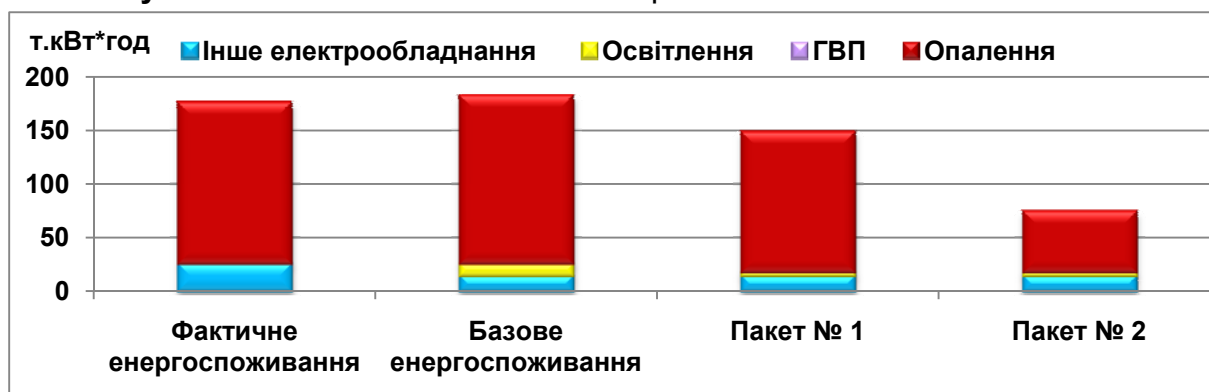
Рисунок 8.1. Баланс споживання енергії
