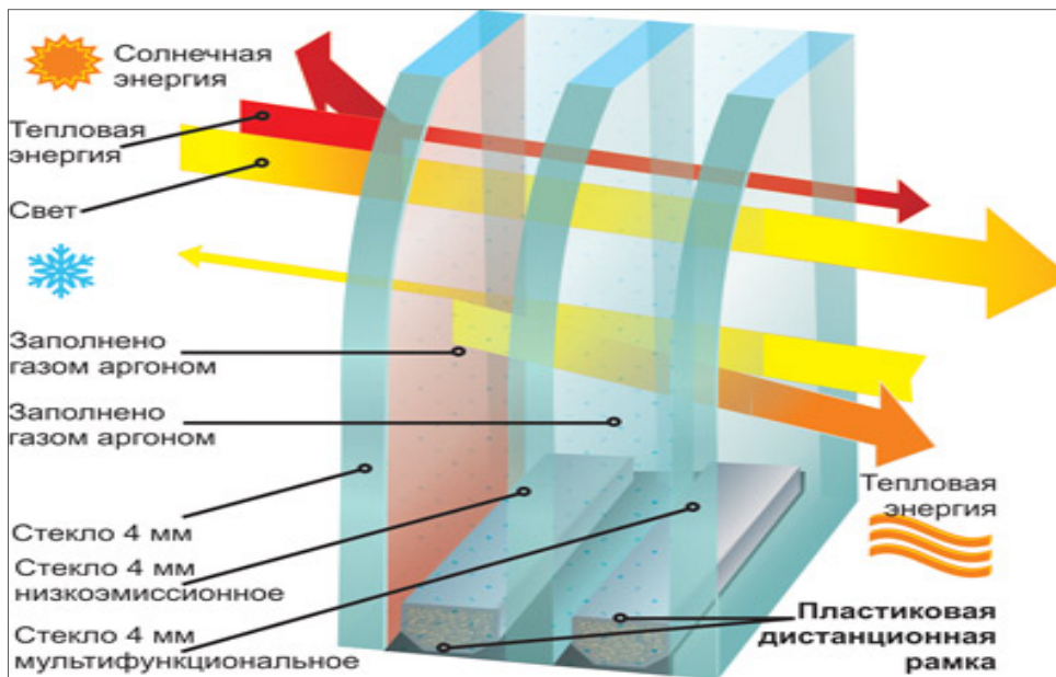
Рисуюнок 7.1.6. Енергозберігаючий склопакет
