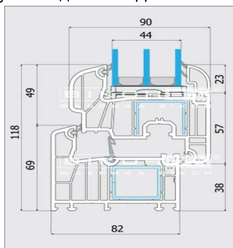
Рисунок 7.1.5. Віконна система типу «Віконда КОТЕДЖ».
