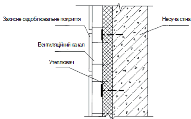
Рисунок 7.1.3. Утеплення стін за методом «керамічний вентиляований фасад»
