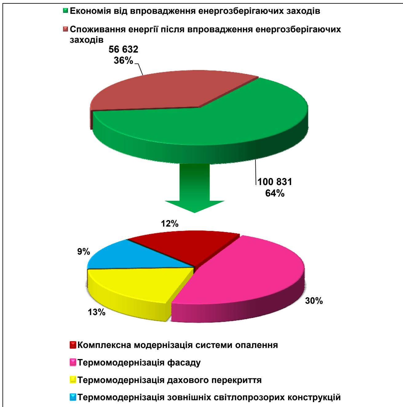
Рисунок 7.2. Баланс економії спожитої енергії будівлею, кВт*год/рік
