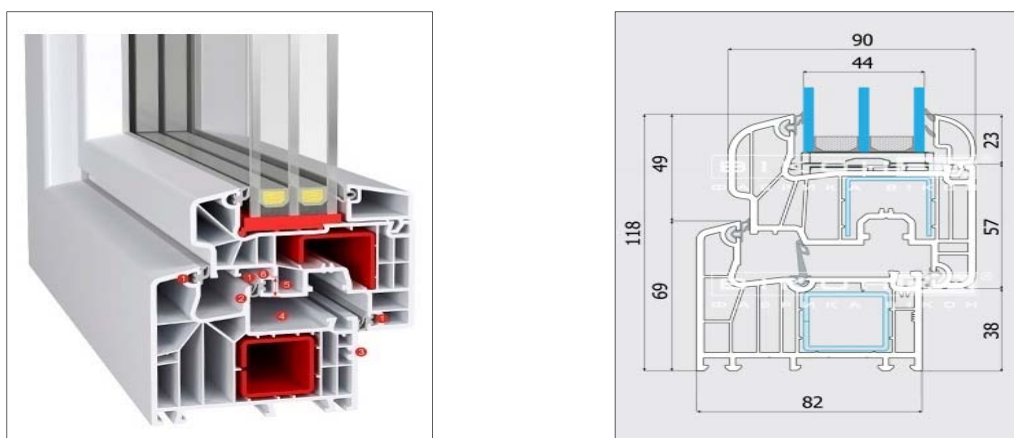
Рисунок 7.1.5. Віконна система типу «Віконда КОТЕДЖ».
