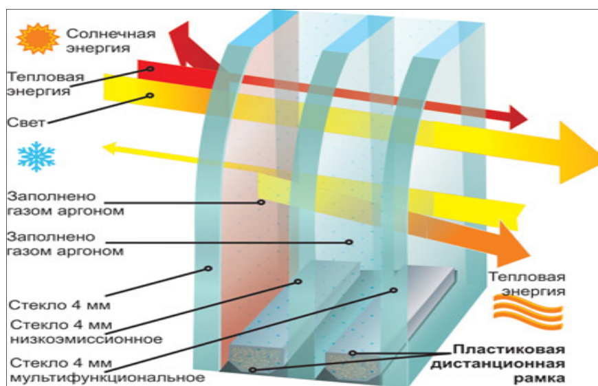
Рисунок 7.1.6. Енергозберігаючий склопакет
