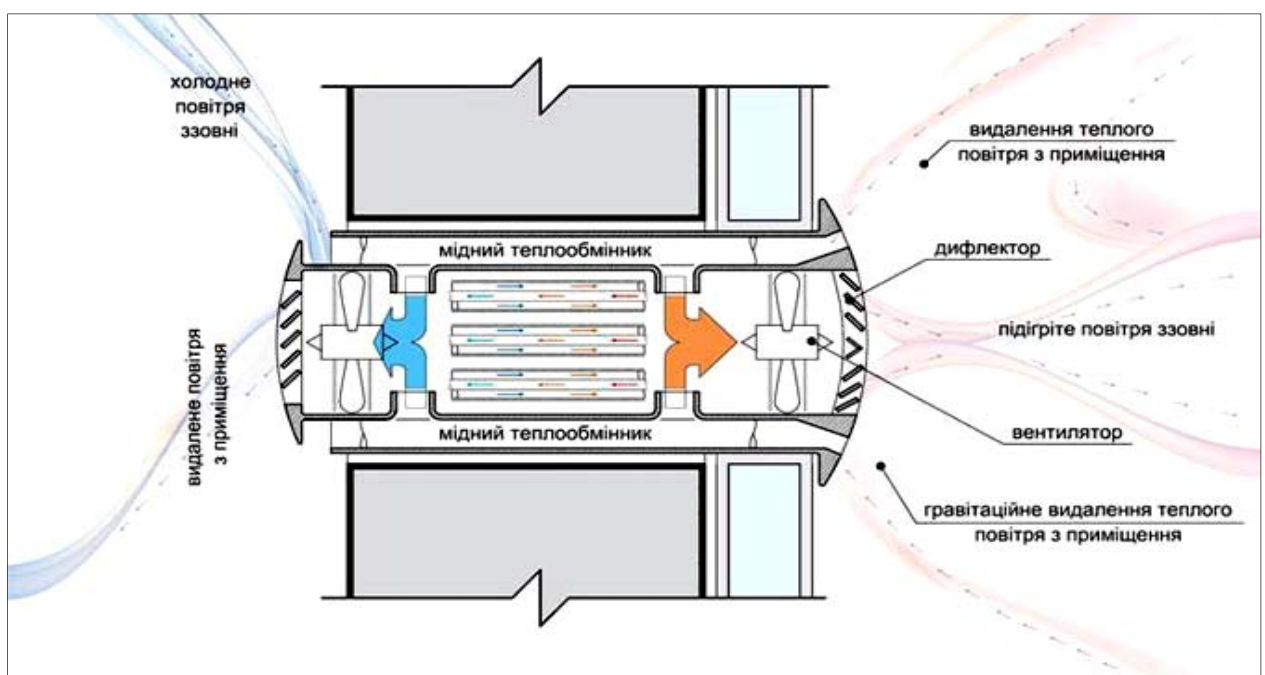
Рисунок 7.1.7. Схема децентралізованої системи вентиляції типу Прана
