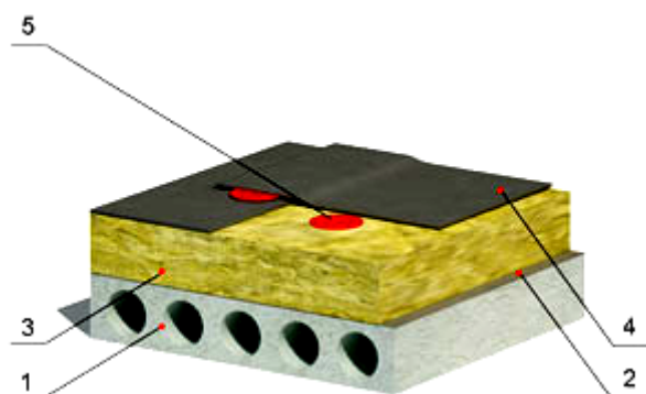
Рисунок 7.1.4. Структура утеплення дахового перекриття
