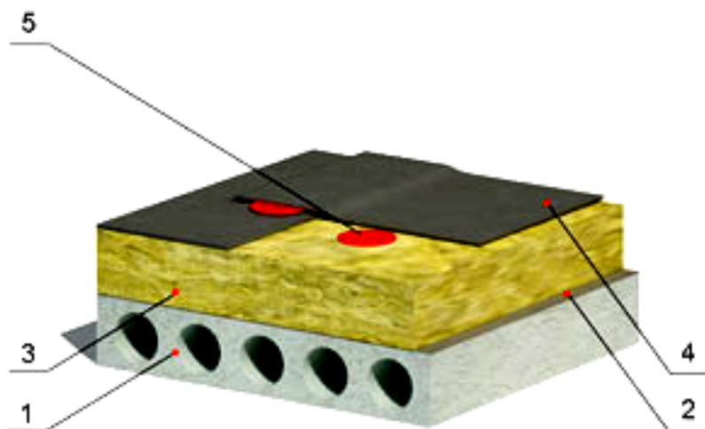
Рисунок 7.1.6. Структура утеплення дахового перекриття
