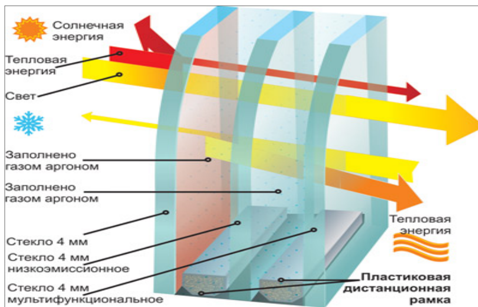
Рисунок 7.1.9. Енергозберігаючий склопакет
