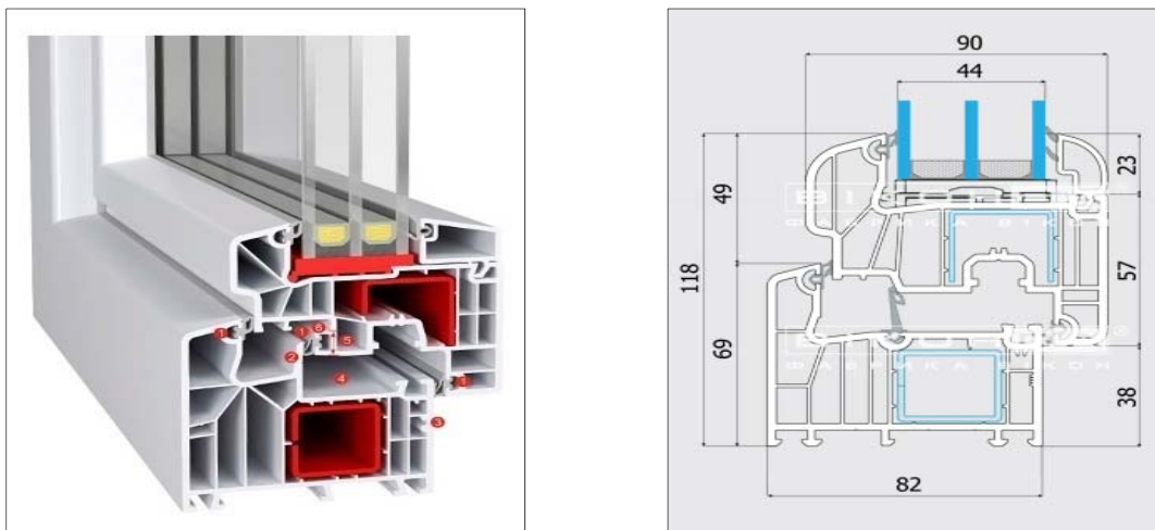
Рисунок 7.1.8. Віконна система типу «Віконда КОТЕДЖ».
