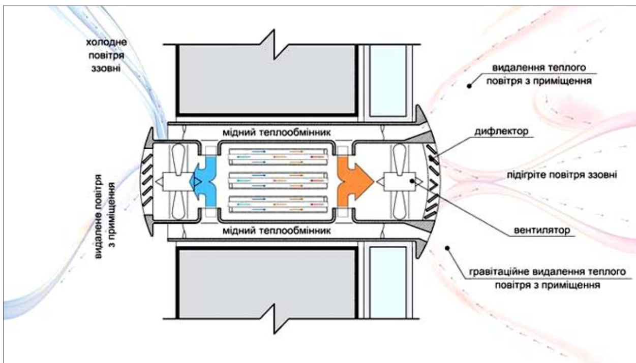
Рисунок 7.1.10. Схема децентралізованої системи вентиляції типу Прана
