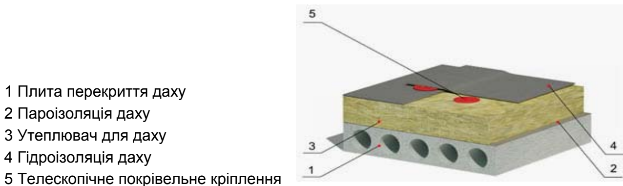
Рисунок 7.1.4. Структура утеплення даху
