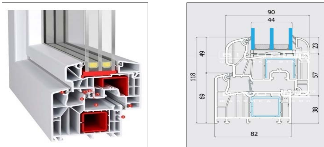
Рисунок 7.1.6. Віконна система типу «Віконда КОТЕДЖ».
