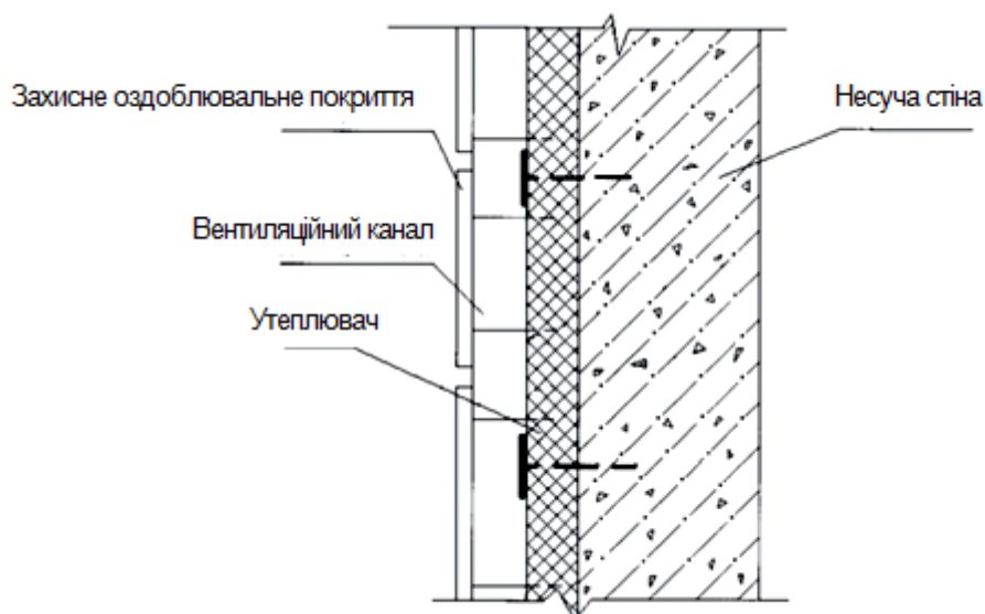
Рисунок 7.1.3. Утеплення стін за методом «керамічний вентиляований фасад»
