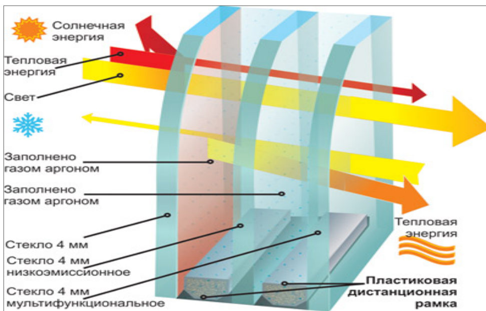
Рисунок 7.1.7. Енергозберігаючий склопакет
