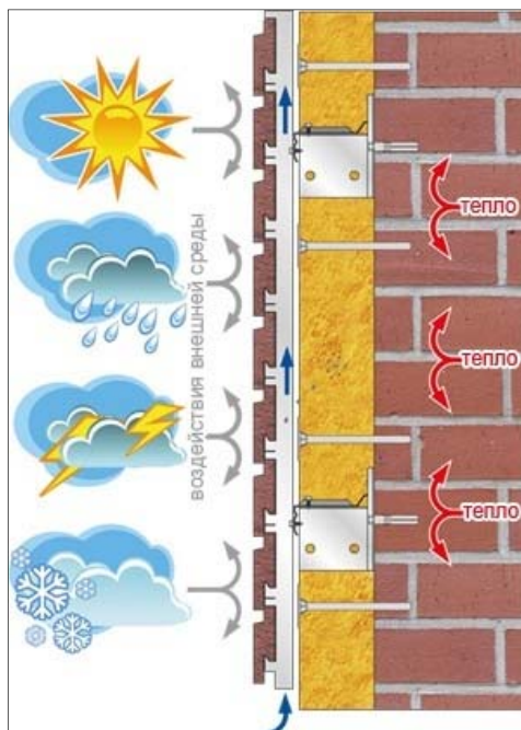
Рисунок. Фасадна система «СКАНРОК»
