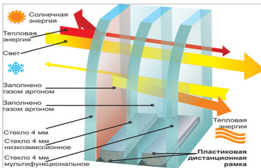
Рисунок 7.1.7. Енергозберігаючий склопакет
