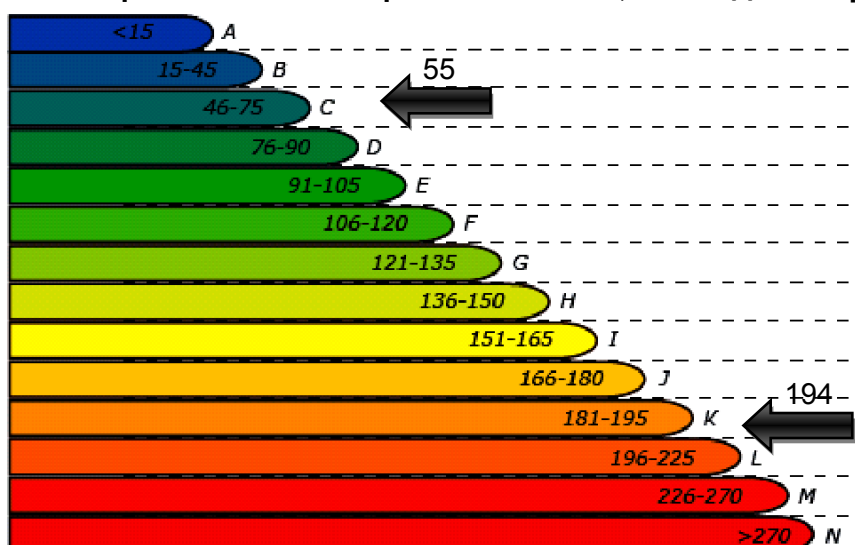
Рисунок 1. Клас енергоефективності будівлі до та після термомодернізації (згідно класифікації енергоефективності будівель в країнах ЄС).
