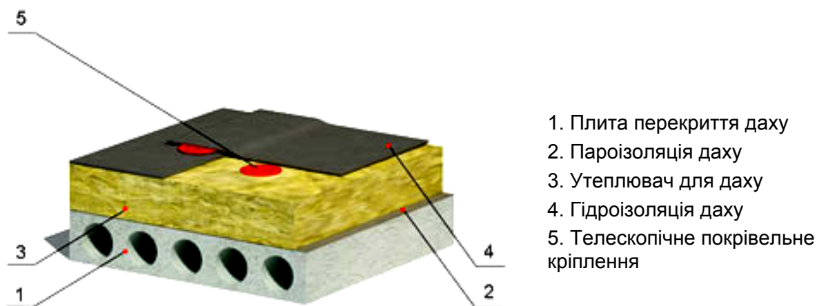
Рисунок 7.1.4. Структура утеплення дахового перекриття
