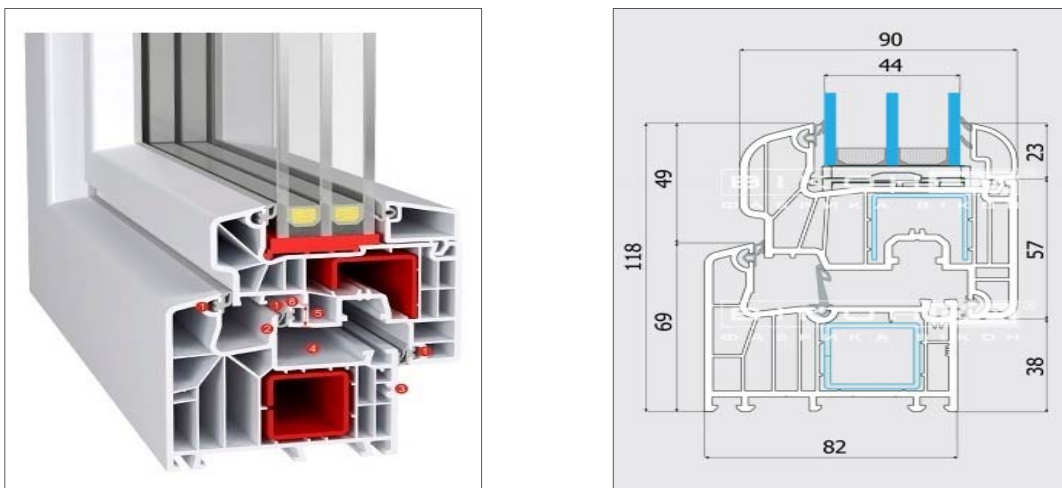
Рисунок 7.1.6. Віконна система типу «Віконда КОТЕДЖ».
