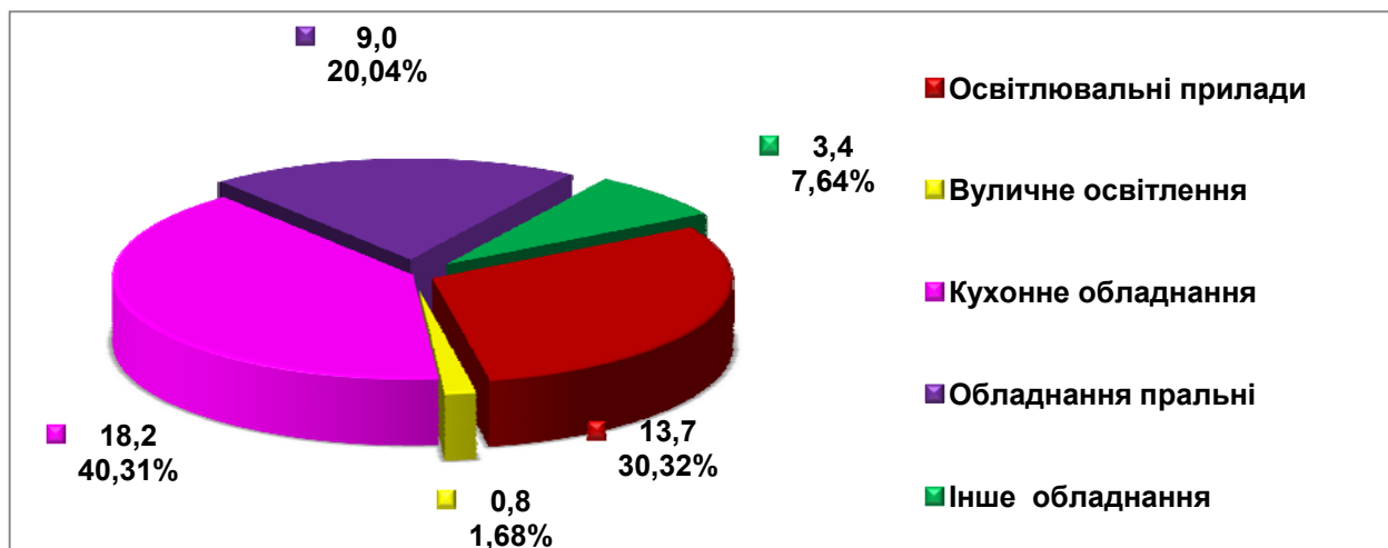
Рисунок 6.2.1. Баланс базового споживання електричної енергії, тис.кВт·год/рік
