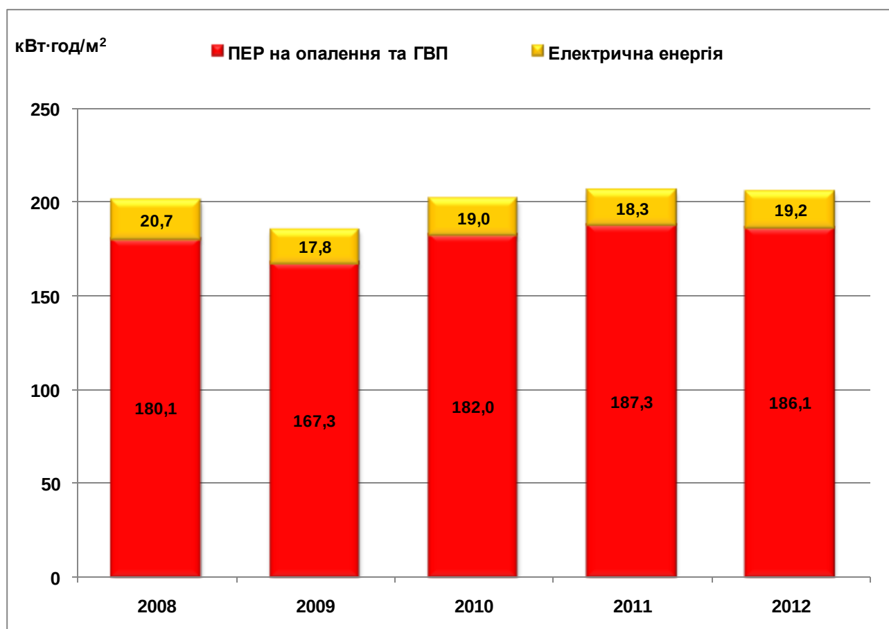
Рисунок 2.9.1. Загальне фактичне питома споживання ПЕР (кВт·год/м 2 в рік)
