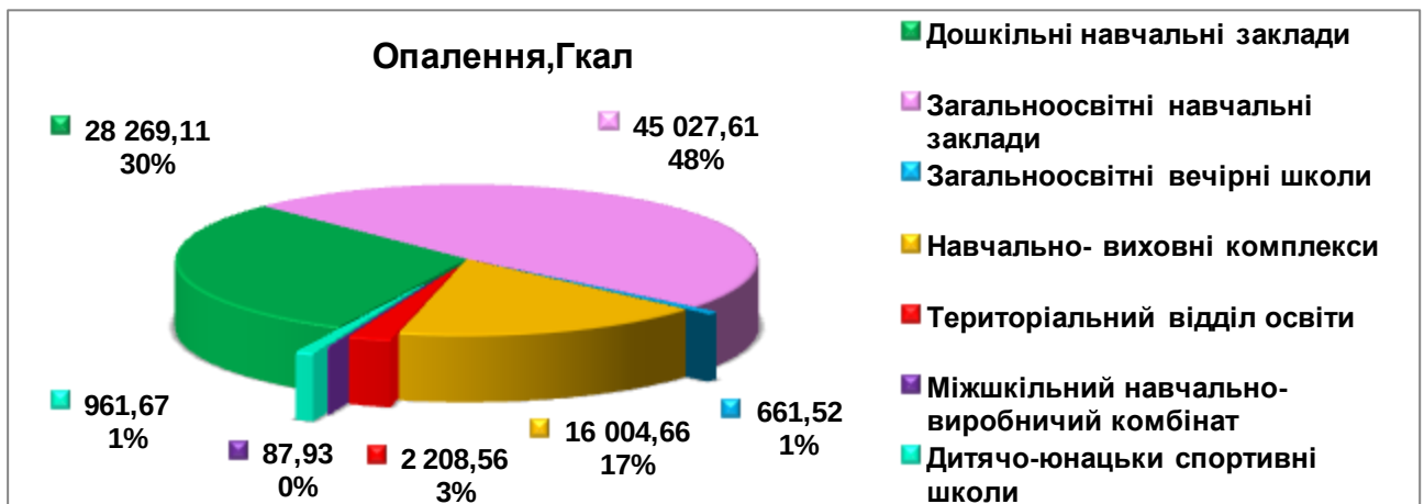
Рисунок 2.3.4. Споживання теплової енергії на опалення з розподілом по галузях за 2012 рік
