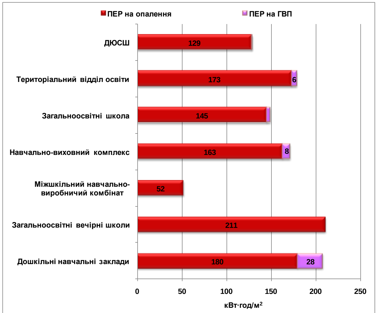
Рисунок 2.9.2. Фактичне питоме споживання ПЕР на опалення та ГВП
